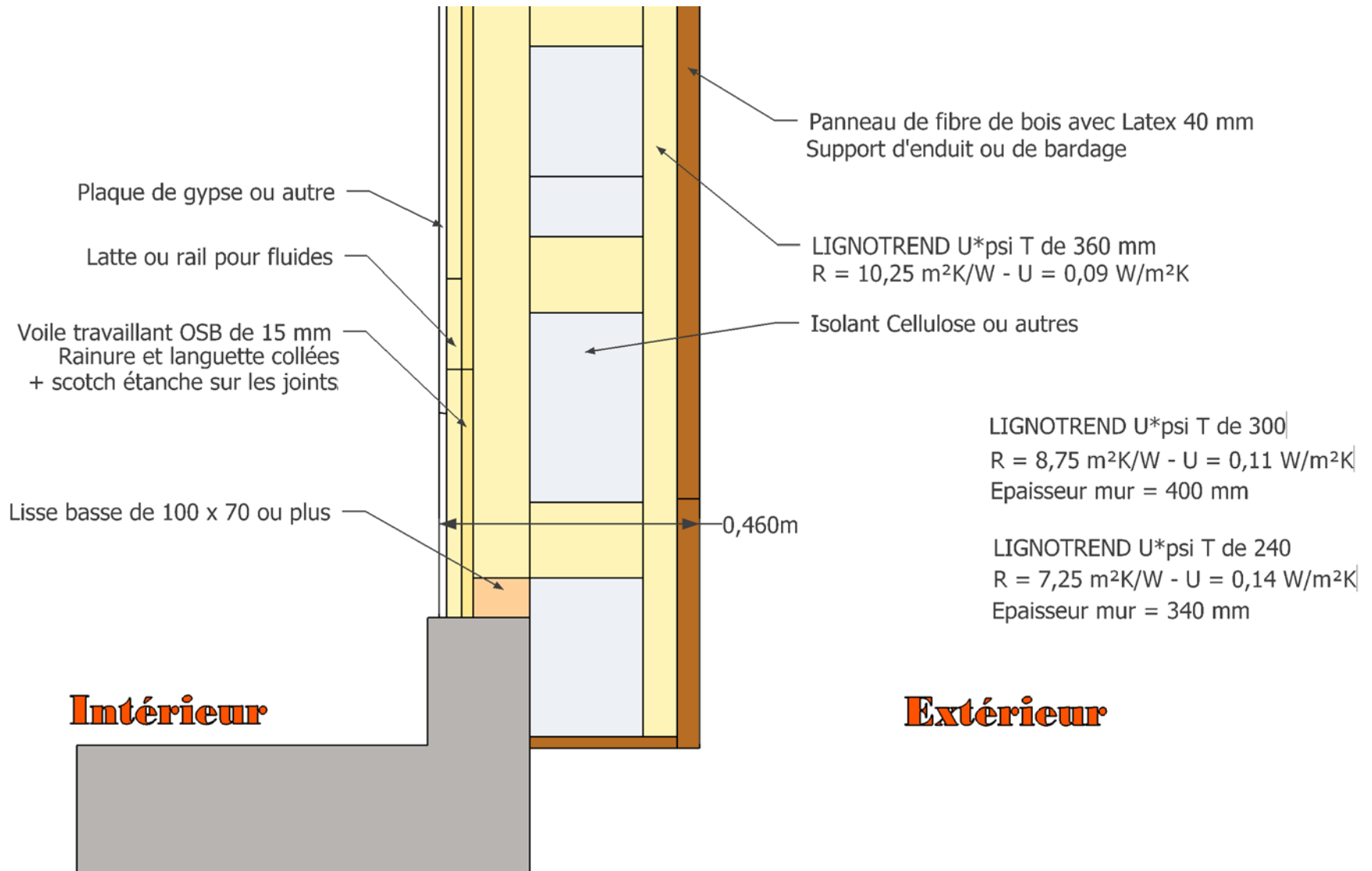
Coupe de principe sur mur passif LIGNOTREND U*psi 360
