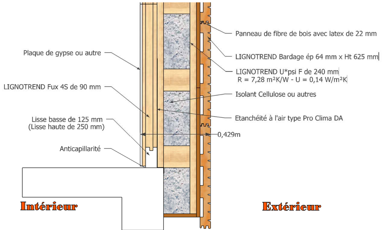
Coupe de principe sur mur passif LIGNOTREND Fux 4S + U*psi F240 + Bardage
