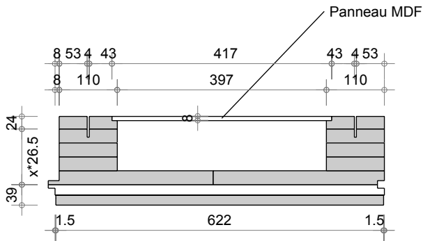
HBV Q2 Z1 Joint creux de 3mm
