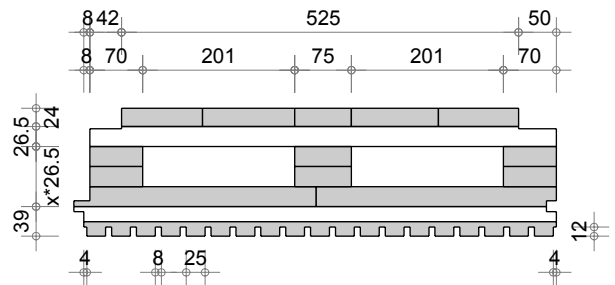
Bloc Q3 Acoustique alpha Z1 (625-25-8)
