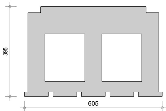
Acoustique Q3 classique 395 BV
