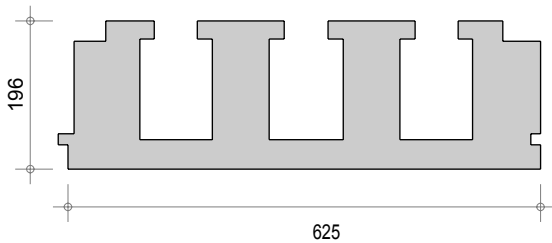
Dalle R Q4 249
