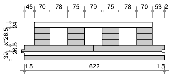
Dalle D Q4 alpha Z1 (625-12-4, P.: 12mm)
