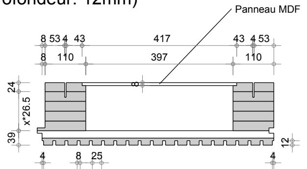
HBV Q2 alpha (625-25-8, Profondeur: 12mm)
