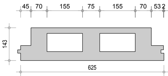
Dalle D Q3 196
