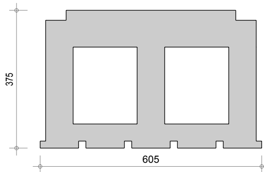
Acoustique Q3 classique 375 BV
