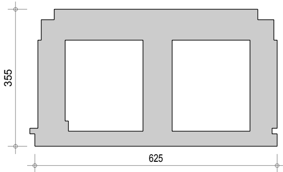
Bloc Q3 BV 395
