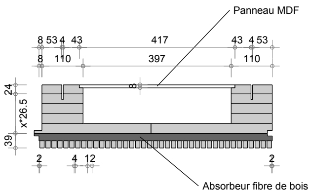
HBV Q2 Acoustique alpha Z1 (625-12-4)
