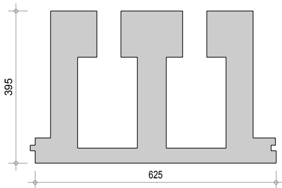
Dalle R Q3 BV 395
