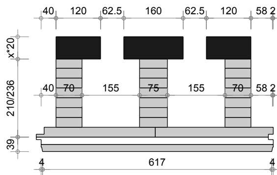
Dalle R Q3 Z1 BV Joint V de 7,9mm
