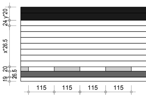
Acoustique Q3 classique BV coupe long.
