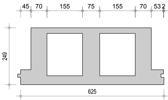
Dalle D Q3 249
