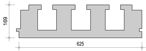
Dalle R Q4 222
