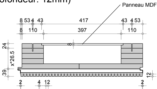
HBV Q2 alpha Z1 (625-12-4, Profondeur: 12mm)
