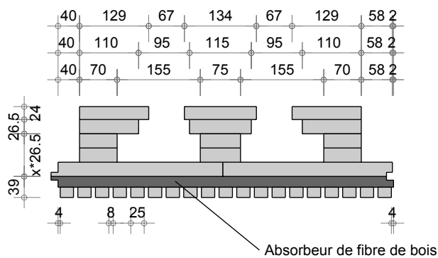
Dalle R Q3 Acoustique alpha Z1 (625-25-8)
