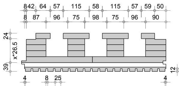
Dalle R Q4 Acoustique alpha Z1 (625-25-8)
