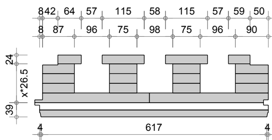
Dalle R Q4 alpha Z1 (625-25-8, Profondeur: 12mm)
