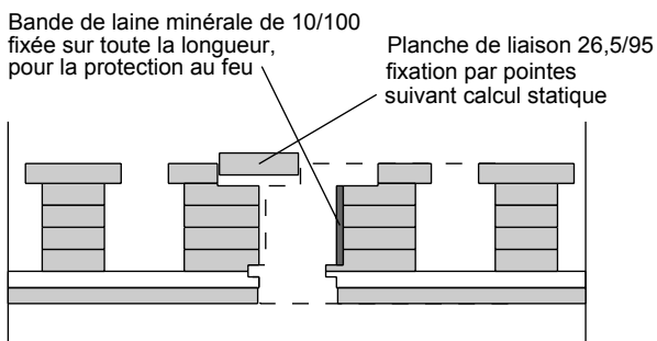
Dalle R Q4 pièce de liaison
