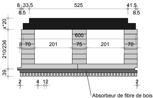
Bloc Q3 Acoustique alpha Z1 BV (625-12-4)
