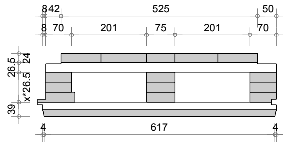
Bloc Q3 alpha (625-25-8, Profondeur: 12mm)
