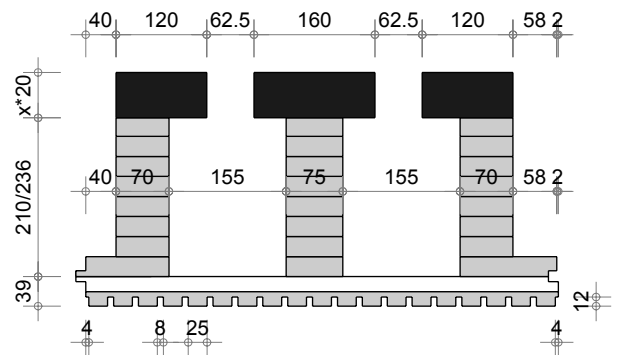
Dalle R Q3 alpha BV (625-25-8, P.: 12mm)
