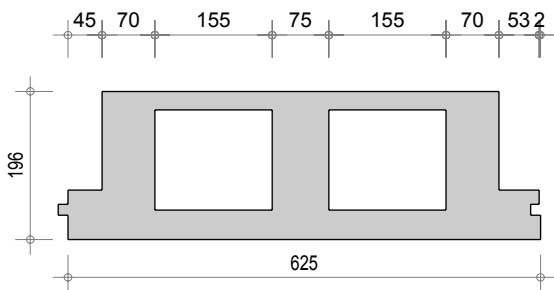
Dalle D Q3 249
