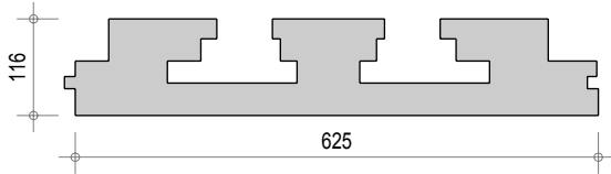
Dalle R Q3 169
