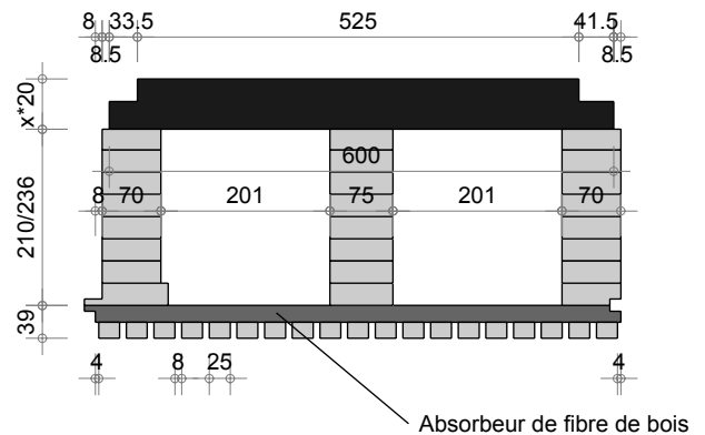
Bloc Q3 Acoustique alpha BV (625-25-8)
