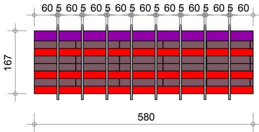
Coupe Transversale Type 60/160
