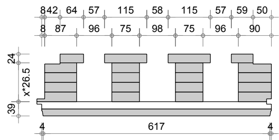
Dalle R Q4 alpha (625-25-8, Profondeur: 12mm)
