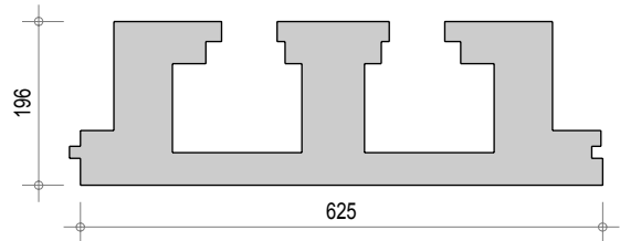
Dalle R Q3 249
