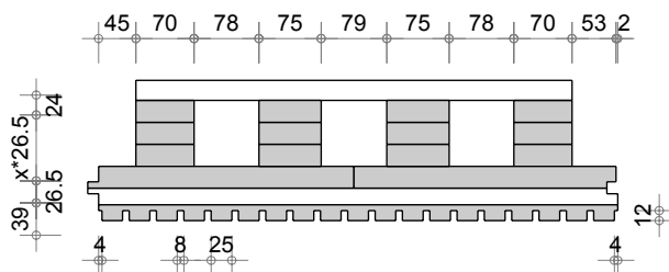
Dalle D Q4 Acoustique alpha Z1 (625-25-8)
