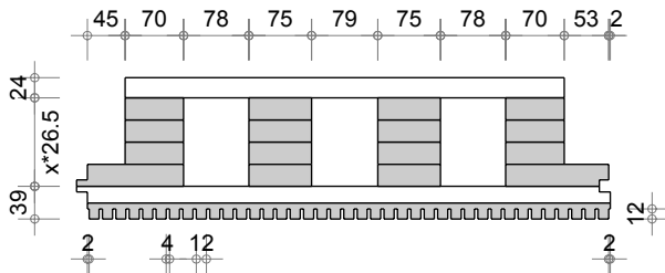
Dalle D Q4 pièce de liaison
