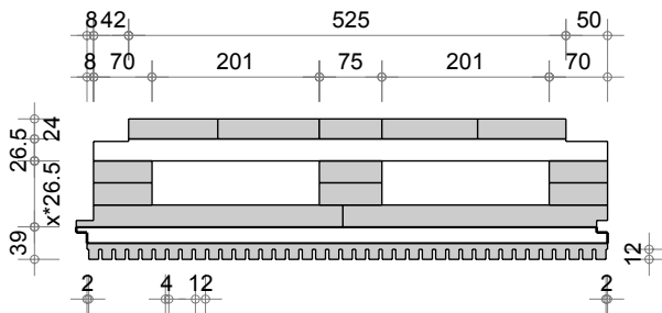
Bloc Q3 Acoustique alpha Z1 (625-12-4)
