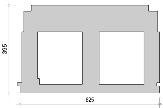
Bloc Q3 BV 395
