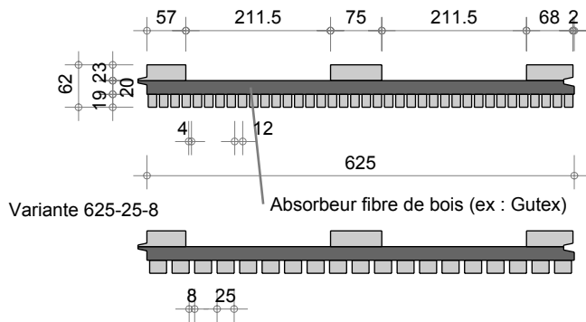
Détail de montage sous dalle ech. 1:7
