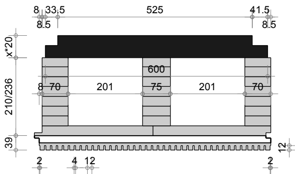
Bloc Q3 alpha Z1 BV (625-12-4, P.: 12mm)
