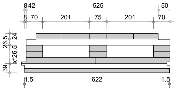
Bloc Q3 alpha Z1 (625-12-4, Profondeur: 12mm)
