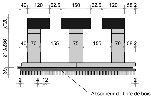
Dalle R Q3 Acoustique BV coupe long.
