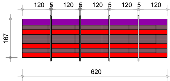
Coupe Transversale Type 120/160
