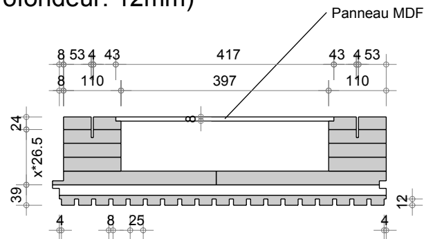
HBV Q2 alpha Z1 (625-25-8, Profondeur: 12mm)
