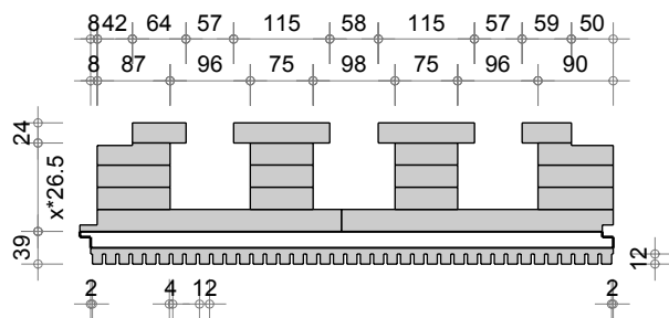
Dalle R Q4 Acoustique alpha Z1 (625-12-4)
