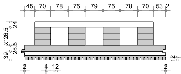
Dalle D Q4 Acoustique alpha Z1 (625-12-4)
