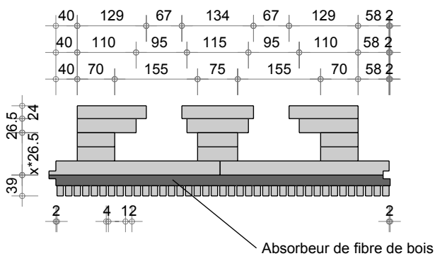
Dalle R Q3 Acoustique coupe long.
