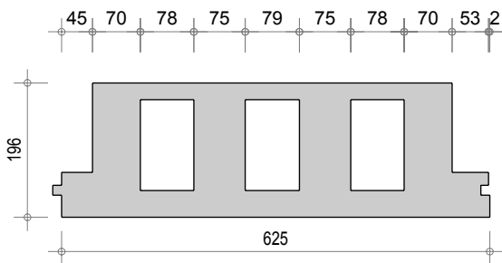
Dalle D Q4 249
