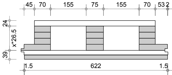
Dalle D Q3 alpha (625-12-4, P.: 12mm)
