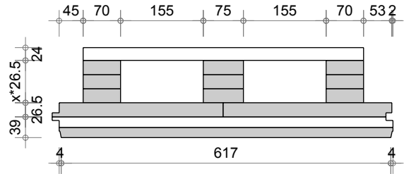
Dalle D Q3 alpha Z1 (625-25-8, P.: 12mm)
