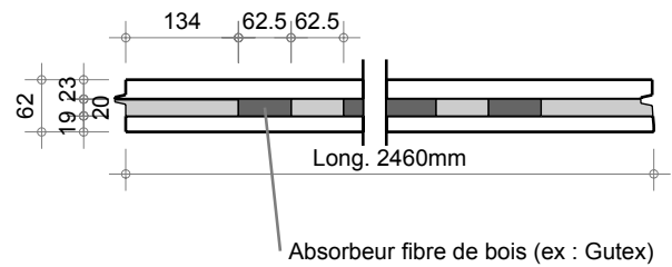
Coupe longitudinale ech. 1:10
