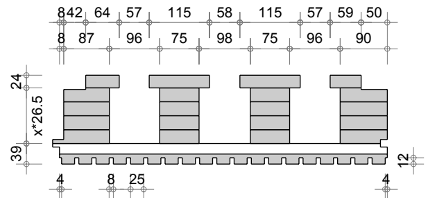
Dalle R Q4 Acoustique alpha (625-25-8)
