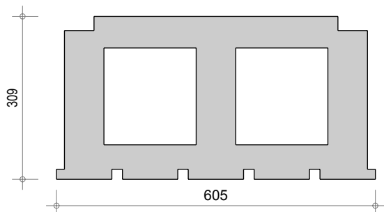
Acoustique Q3 classique 355 BV
