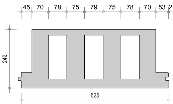
Dalle D Q4 249
