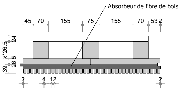
Dalle D Q3 Acoustique coupe long.
