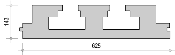
Dalle R Q3 196
