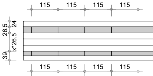
Bloc Q3 pièce de liaison
