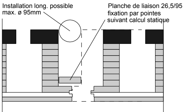
Dalle R Q3 BV pièce de liaison
