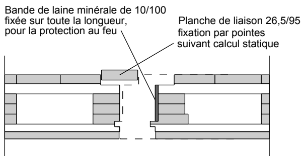
Bloc Q3 pièce de liaison
