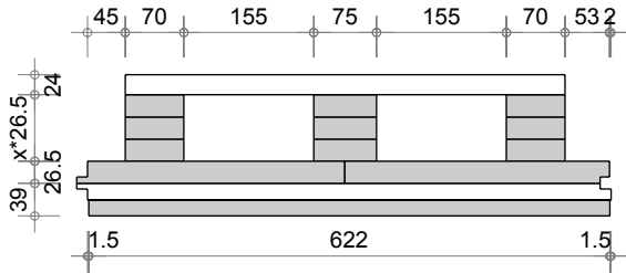
Dalle D Q3 alpha Z1 (625-12-4, P.: 12mm)
