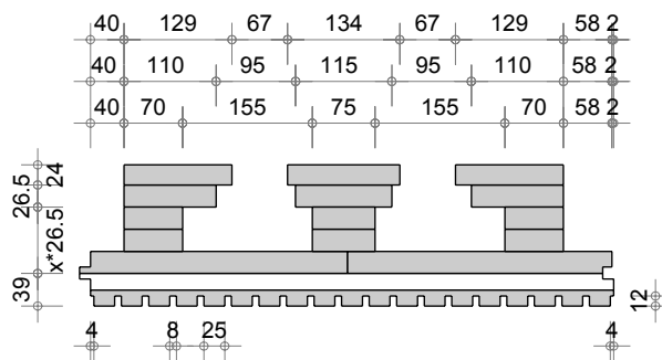
Dalle R Q3 Acoustique alpha Z1 (625-25-8)
