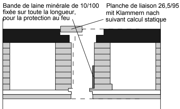
Bloc Q3 BV Pièce de liaison
