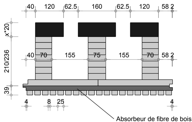
Dalle R Q3 Ac. alpha Z1 BV (625-25-8)
