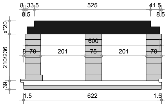
Bloc Q3 BV Joint creux de 3mm
