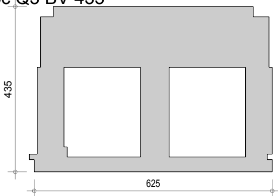
Bloc Q3 BV 435
