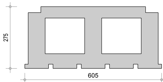
Acoustique Q3 classique 335 BV
