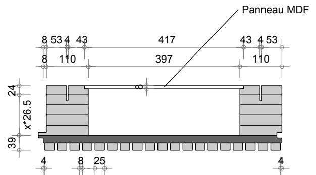
HBV Q2 Acoustique alpha (625-25-8)
