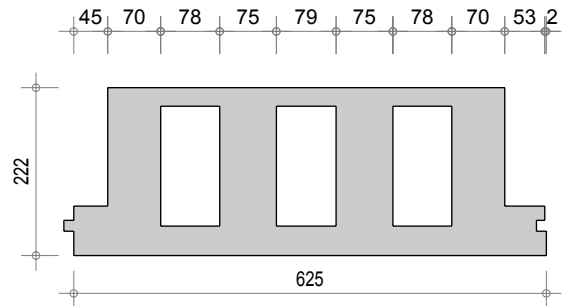
Dalle D Q4 275
