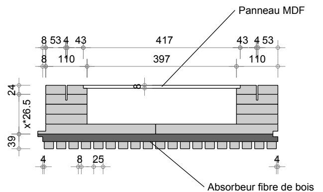
HBV Q2 Acoustique alpha Z1 (625-25-8)
