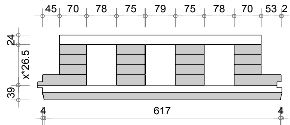
Dalle D Q4 alpha (625-25-8, P.: 12mm)
