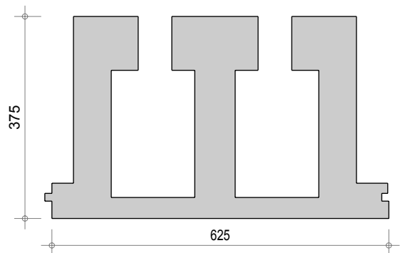
Dalle R Q3 BV 375
