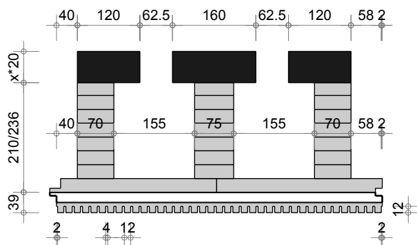
Dalle R Q3 alpha Z1 BV (625-12-4,P.: 12mm)
