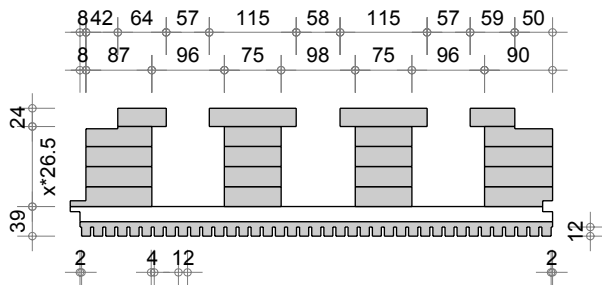
Dalle R Q4 Acoustique alpha (625-12-4)
