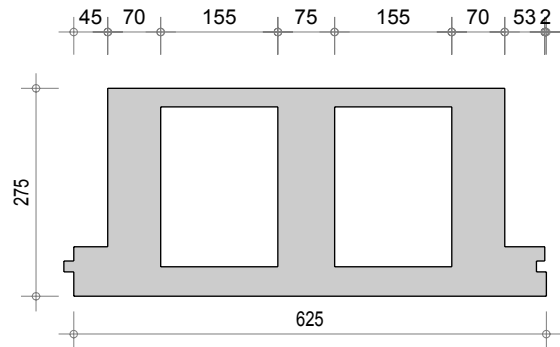
Dalle D Q3 275
