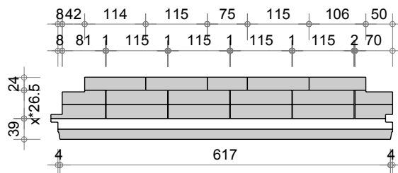
Bloc Q alpha (625-25-8, Profondeur: 12mm)
