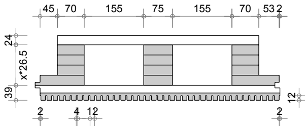
Dalle D Q3 pièce de liaison
