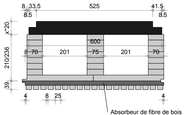
Bloc Q3 Acoustique alpha Z1 BV (625-25-8)
