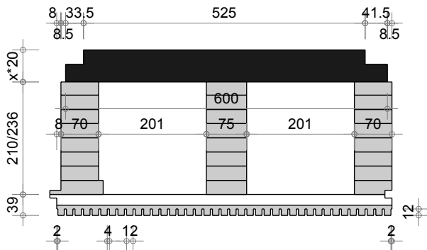
Bloc Q3 alpha BV (625-12-4, P.: 12mm)
