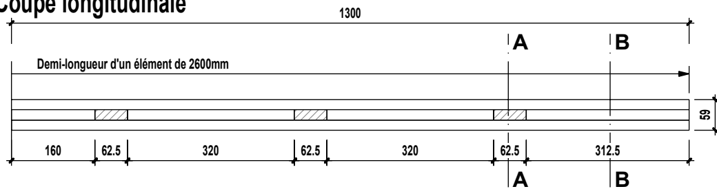
Coupe longitudinale
