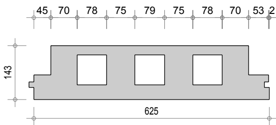
Dalle D Q4 196
