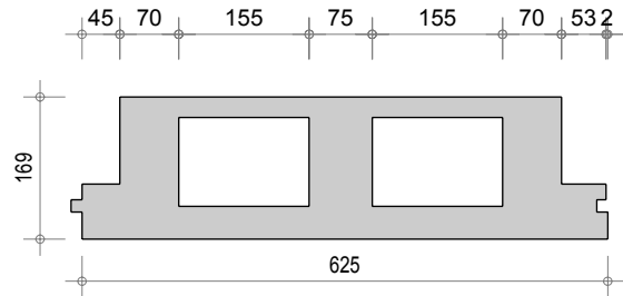
Dalle D Q3 222
