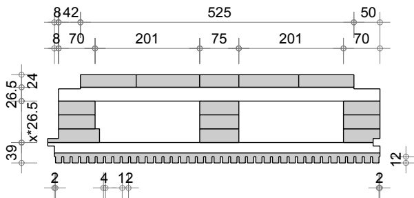
Bloc Q3 Acoustique alpha (625-12-4)
