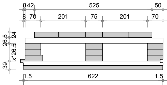
Bloc Q3 alpha (625-12-4, Profondeur: 12mm)
