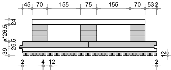
Dalle D Q3 Acoustique alpha Z1 (625-12-4)
