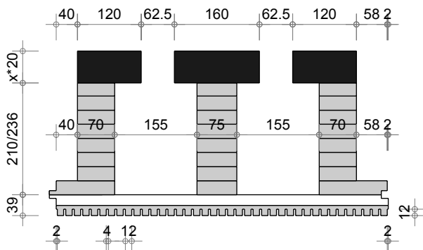
Dalle R Q3 alpha BV (625-12-4, P.: 12mm)
