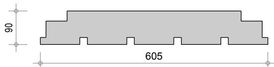
Acoustique Q classique 143
