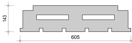
Acoustique Q3 classique 196
