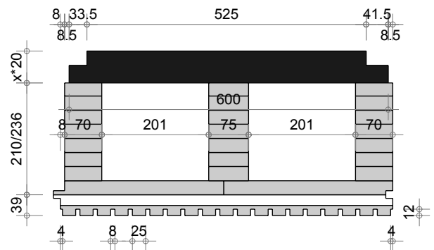
Bloc Q3 alpha Z1 BV (625-25-8, P.: 12mm)
