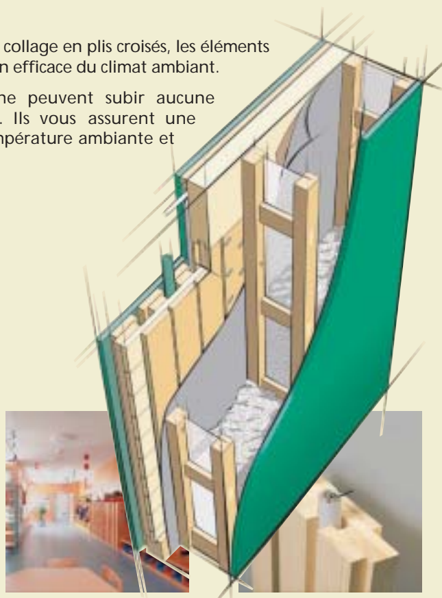
Exemple d'installation de fluides dans les éléments de paroi LIGNOTREND et d'isolation avec U*psi en façade
