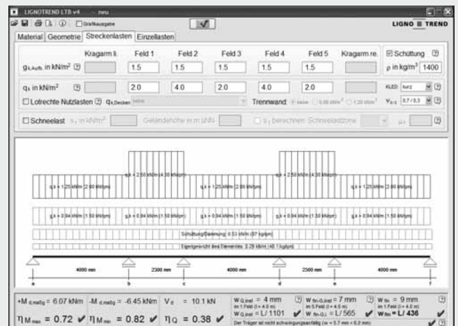
Calcul des systèmes à plusieurs travées (jusqu'à 5 travées) avec concoles.
