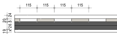
2. Coupe longitudinale LIGNO Acoustique Q classique
