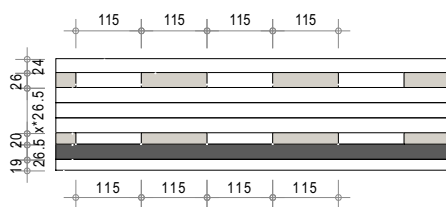
6. Coupe longitudinale LIGNO Acoustique Q3 classique BV
