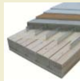
Élément LIGNO HBV (système collaborant bois-béton) avec face acoustique.
